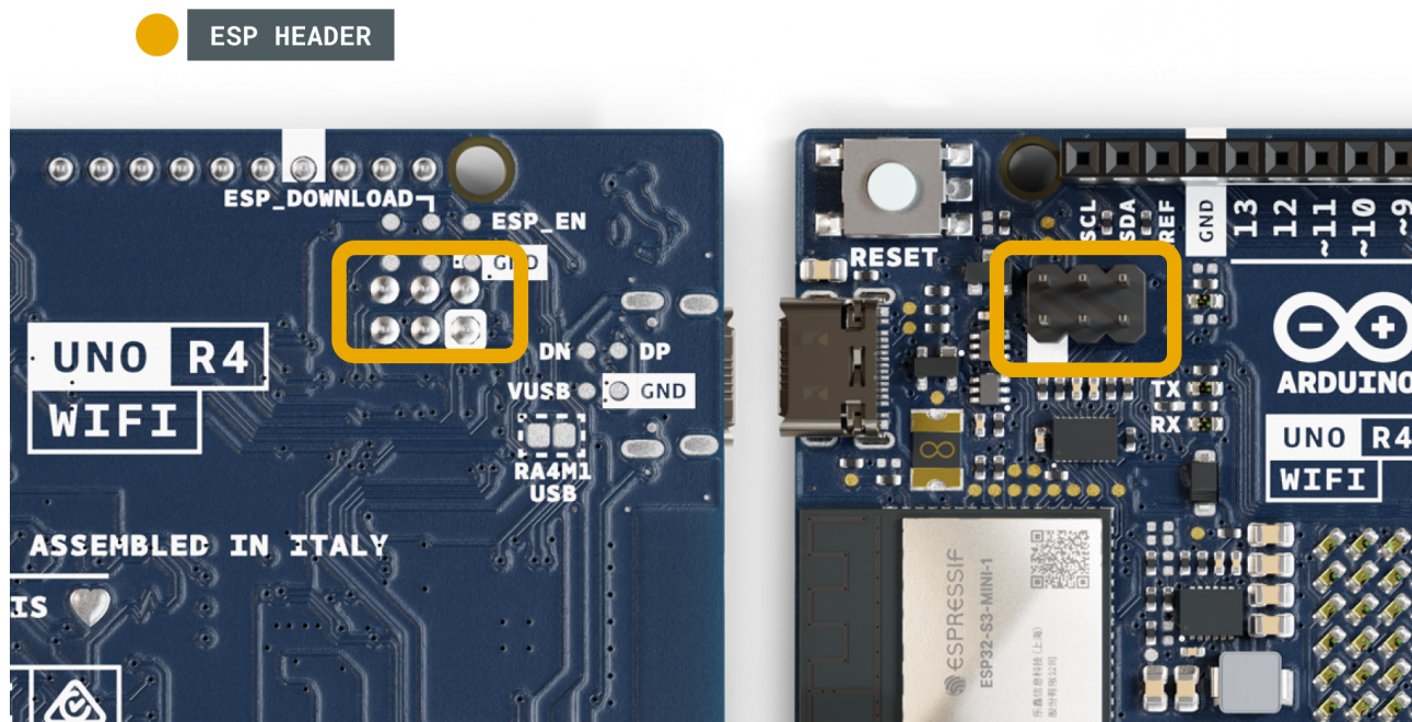
ESP引脚
